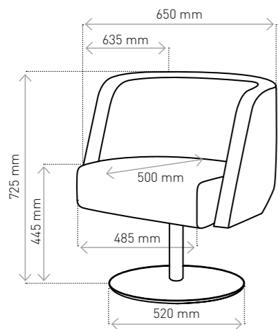
PL Fotel Neon S podstawa płaska obrotowa SK Kreslo Neon S plochý otočný podstavec EN Armchair Neon S flat swivel base CZ Křeslo Neon S plochý otočný podstavec DE Sessel Neon S flacher drehbarer Sockel RU Кресло Neon S плоская поворотная опора
