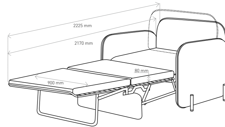
PL Fotel rozkładany Corbu EN Chair bed Corbu DE Ausklappbarer Sessel Corbu
