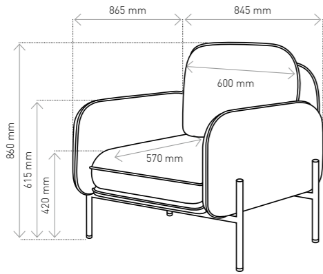
PL Fotel Corbu EN Armchair Corbu DE Sessel Corbu
