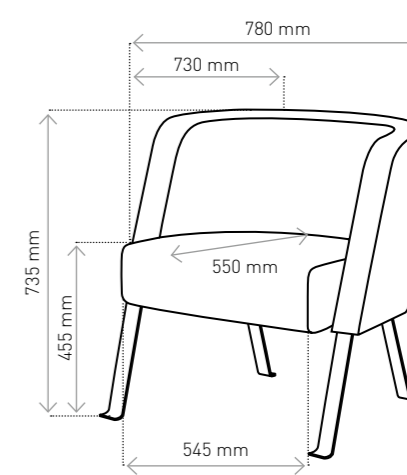
PL Fotel Neon M nóżki metalowe SK Kreslo Neon M kovové nožičky EN Armchair Neon M metal legs CZ Křeslo Neon M kovové nožičky DE Sessel Neon M Metallbeine RU Кресло Neon M металлические ножки
