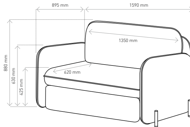
PL Sofa rozkładana Corbu EN Sofa bed Corbu DE Ausklappbares Sofa Corbu
