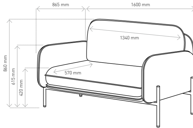
PL Sofa Corbu EN Sofa Corbu DE Sofa Corbu
